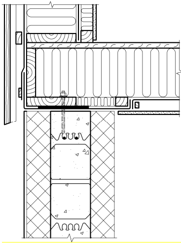
Fig. 5 Eksempel på tilslutning mot etasjeskiller med trebjelkelag.
